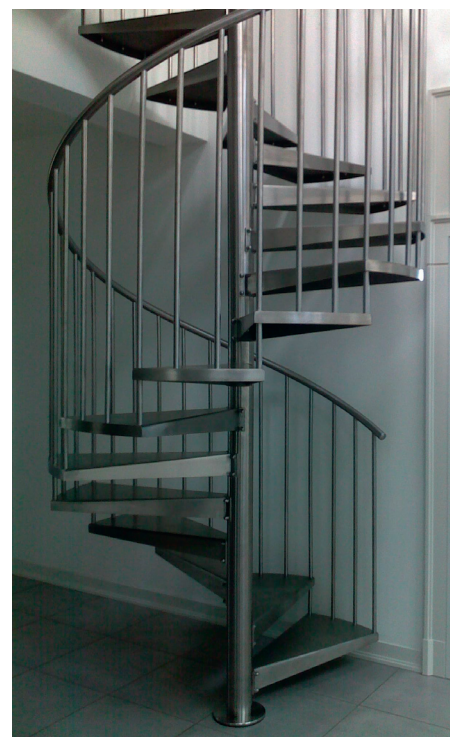
Schody kręcone oraz balustrada ze stali nierdzewnej
